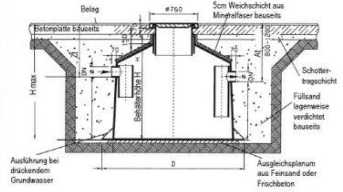
Fettabscheider mit integriertem Schlammfang
